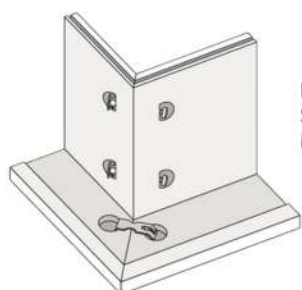
Bisherige Eckverbindung mit Schraubverbindern und Metalleckverbinder.
